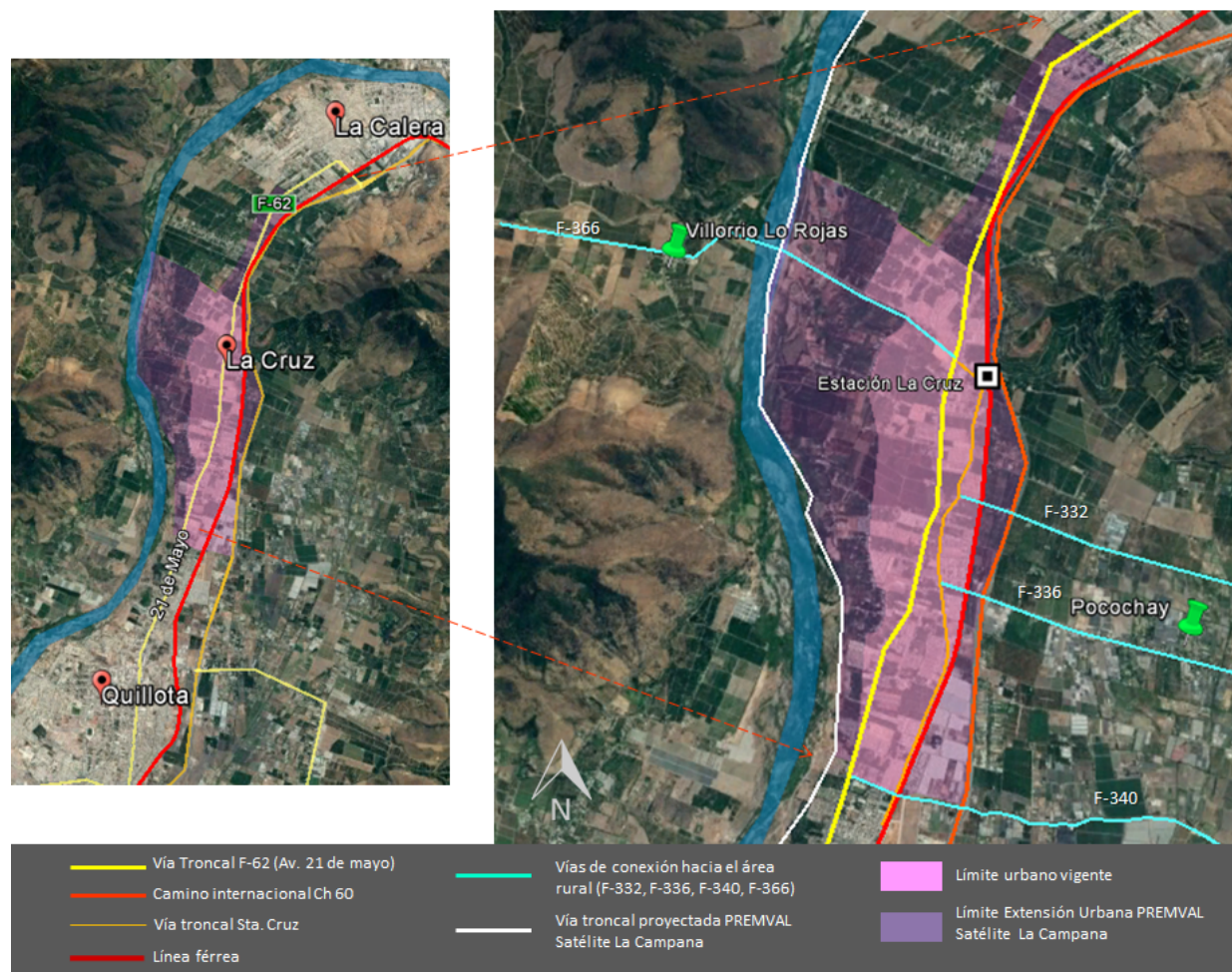
Figura 7-5 Estructuración de la infraestructura de transporte
